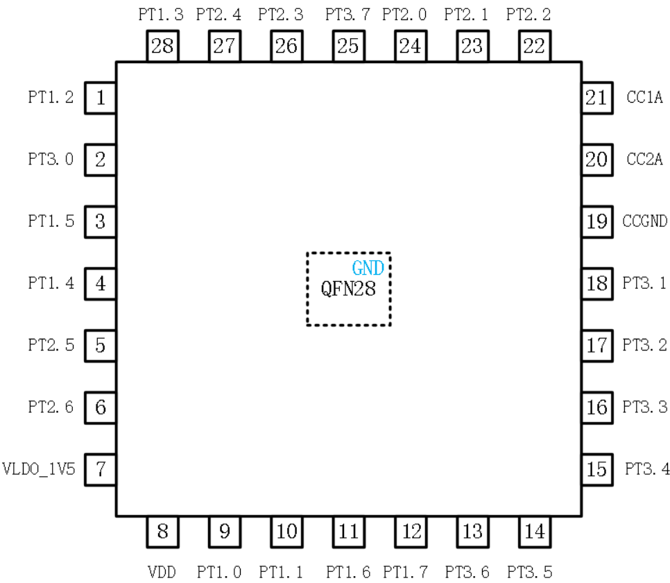
图 1-1 QFN28 管脚图
