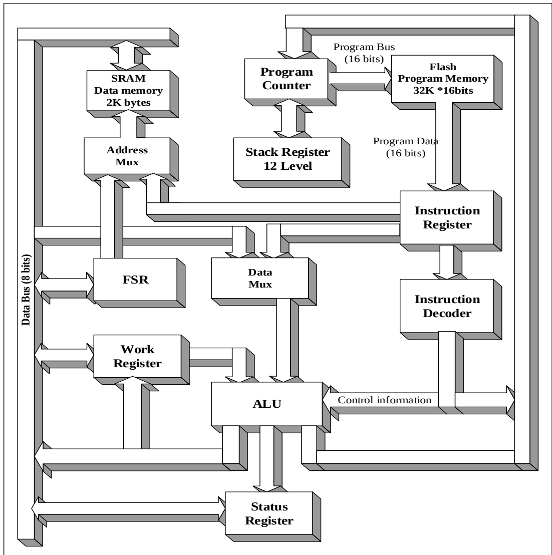
图 2-1 CSU3AF10 CPU 核的功能模块图
