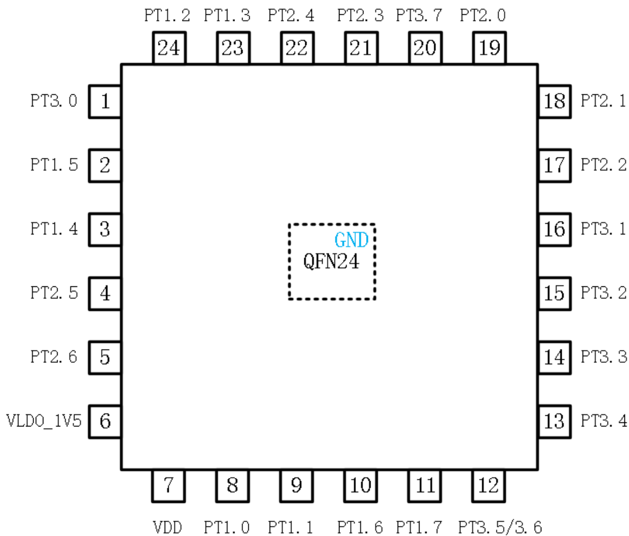
图 1-2 QFN24 管脚图
