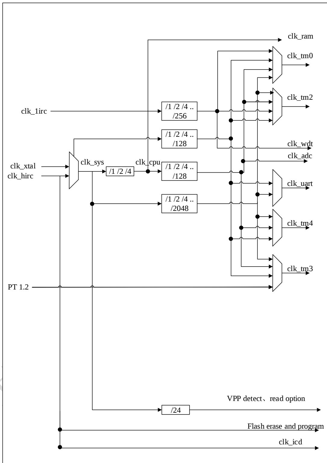
图 2-7 时钟结构
