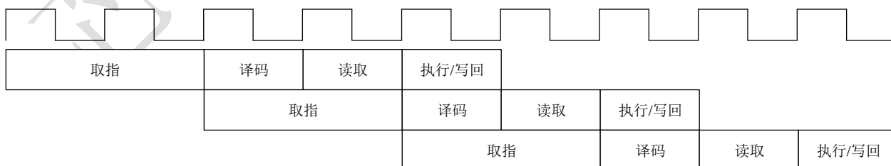
图 2-2 内核流水线
