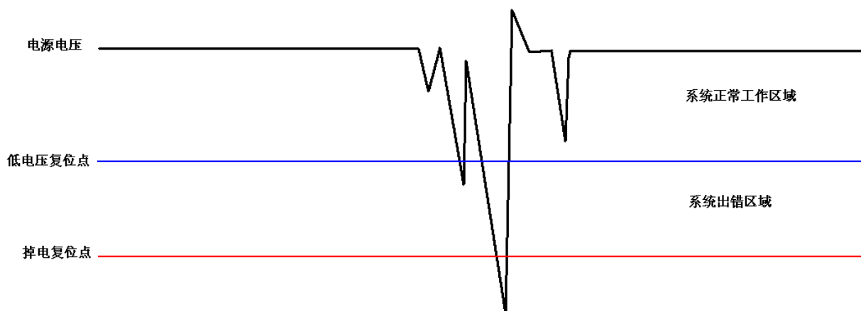
图 2-11 系统掉电复位示意图
