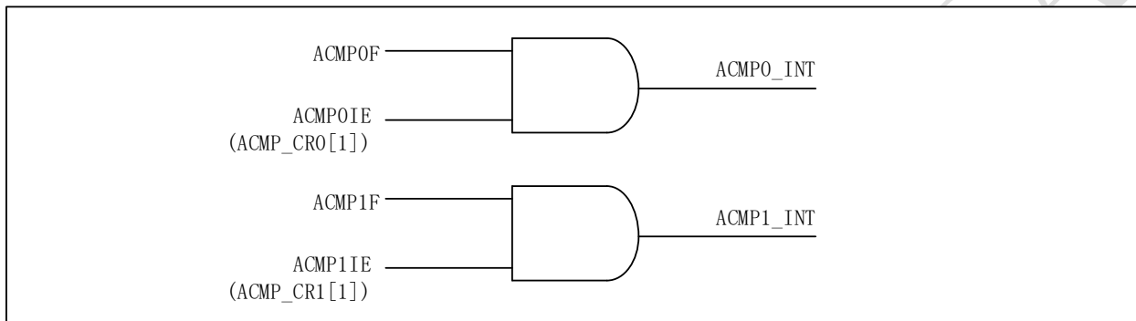
图 3-14 比较器中断源
