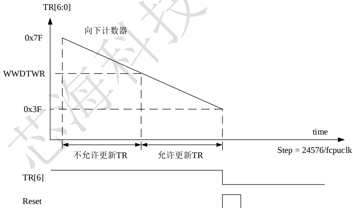
图 3-3 WWDT 时序图
